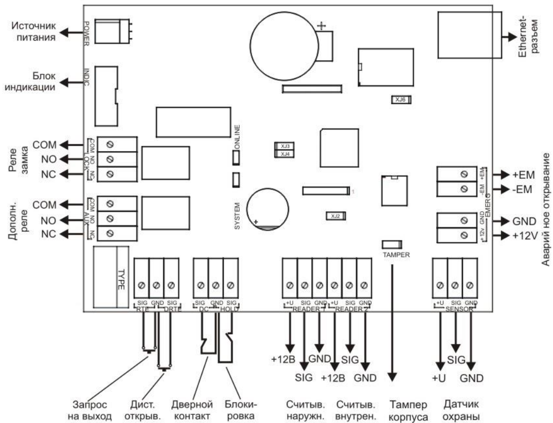
Рисунок 2. Схема платы контроллера NC-2000-IP
