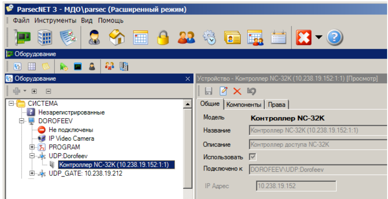
Рисунок 32. Настройка контроллера в ParsecNET 3
