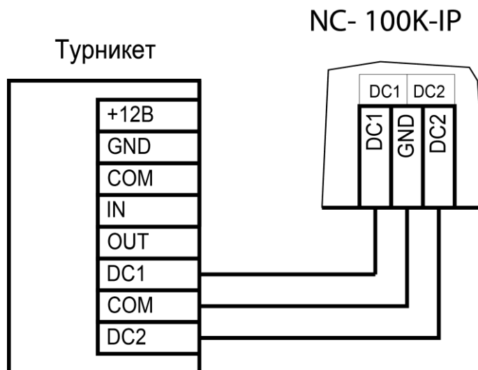
Рисунок 16. Схема подключения турникета с двумя датчиками проворота
