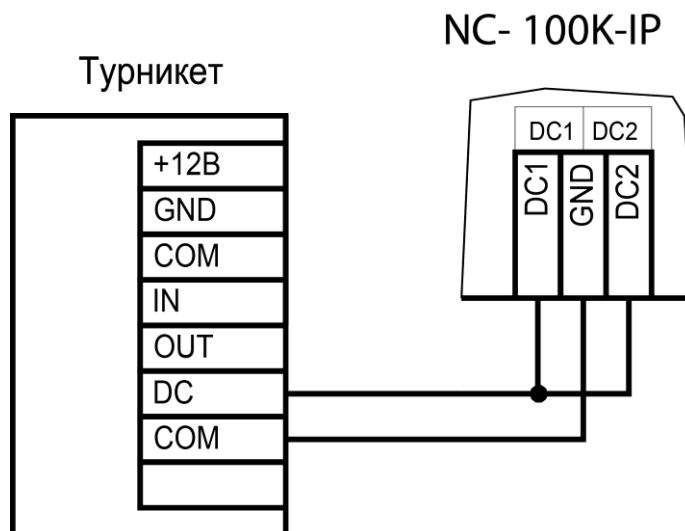
Рисунок 15. Схема подключения турникета с одним датчиком проворота
