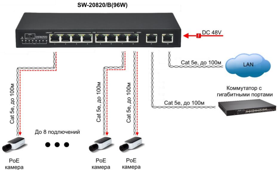
Рис.4 Типовая схема подключения коммутатора SW-20820/B(96W)
