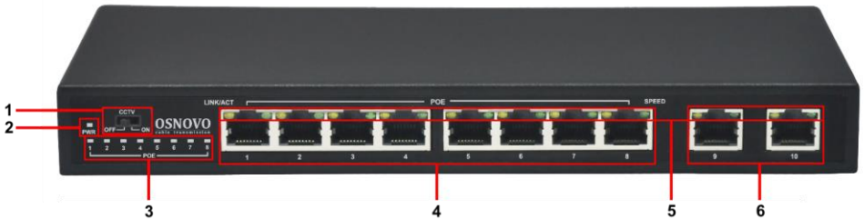
Рис. 2 Коммутатор SW-20820/B(96W), разъемы и индикаторы на передней панели
