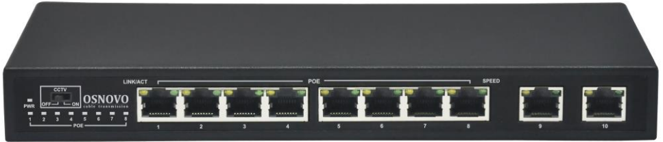
Рис.1 Коммутатор SW-20820/B(96W), внешний вид
