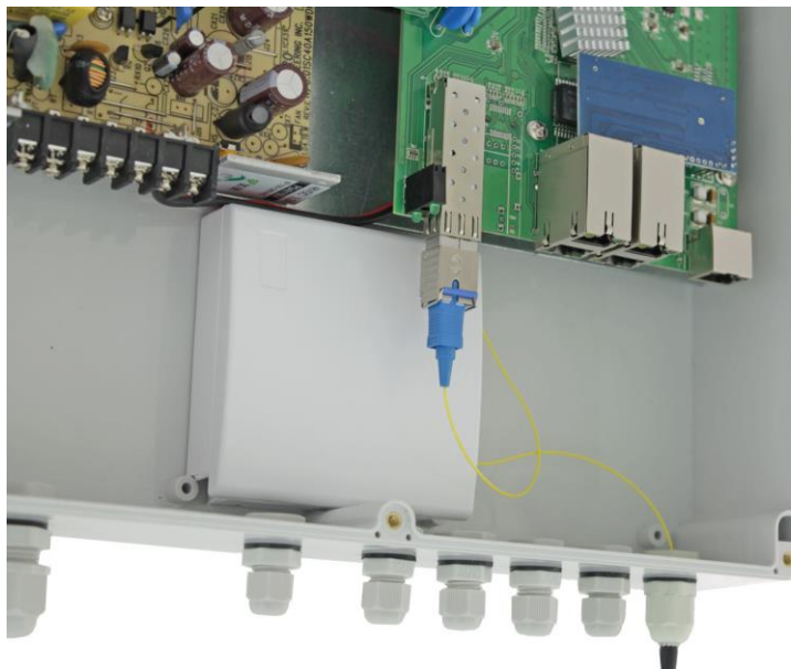
Рис. 5 Коммутатор SW-40501/WC с смонтированным оптическим кроссом (SFP-модуль в комплект поставки не входит)
