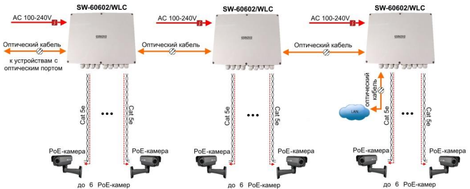
Рис.3.1 Схема применения SW-60602/WLC
