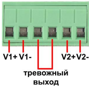
Рис.5.3 Клеммная колодка
