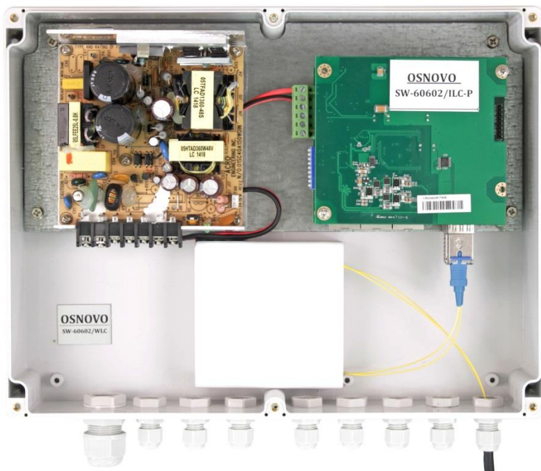
Рис.6.1 Коммутатор со смонтированным оптическим кроссом
