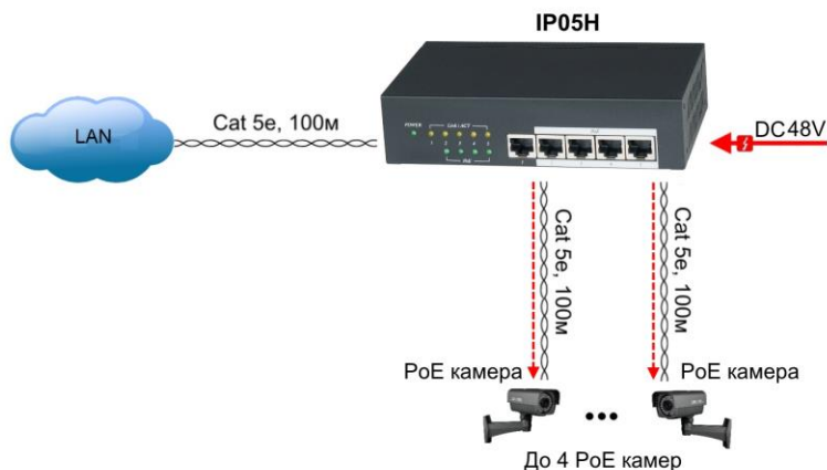
Рис. 3 Схема подключения PoE-коммутатора IP05H
