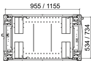
Вид снизу
