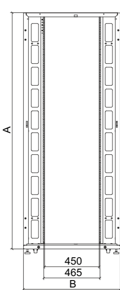
Каркас ШТК-СП-х.8.х
