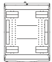
Каркас ШТК-СП-х.8.х
