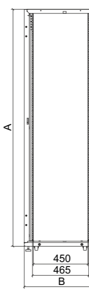
Каркас ШТК-СП-х.6.х
