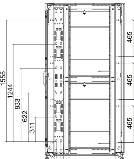
Вид сбоку в разрезе
