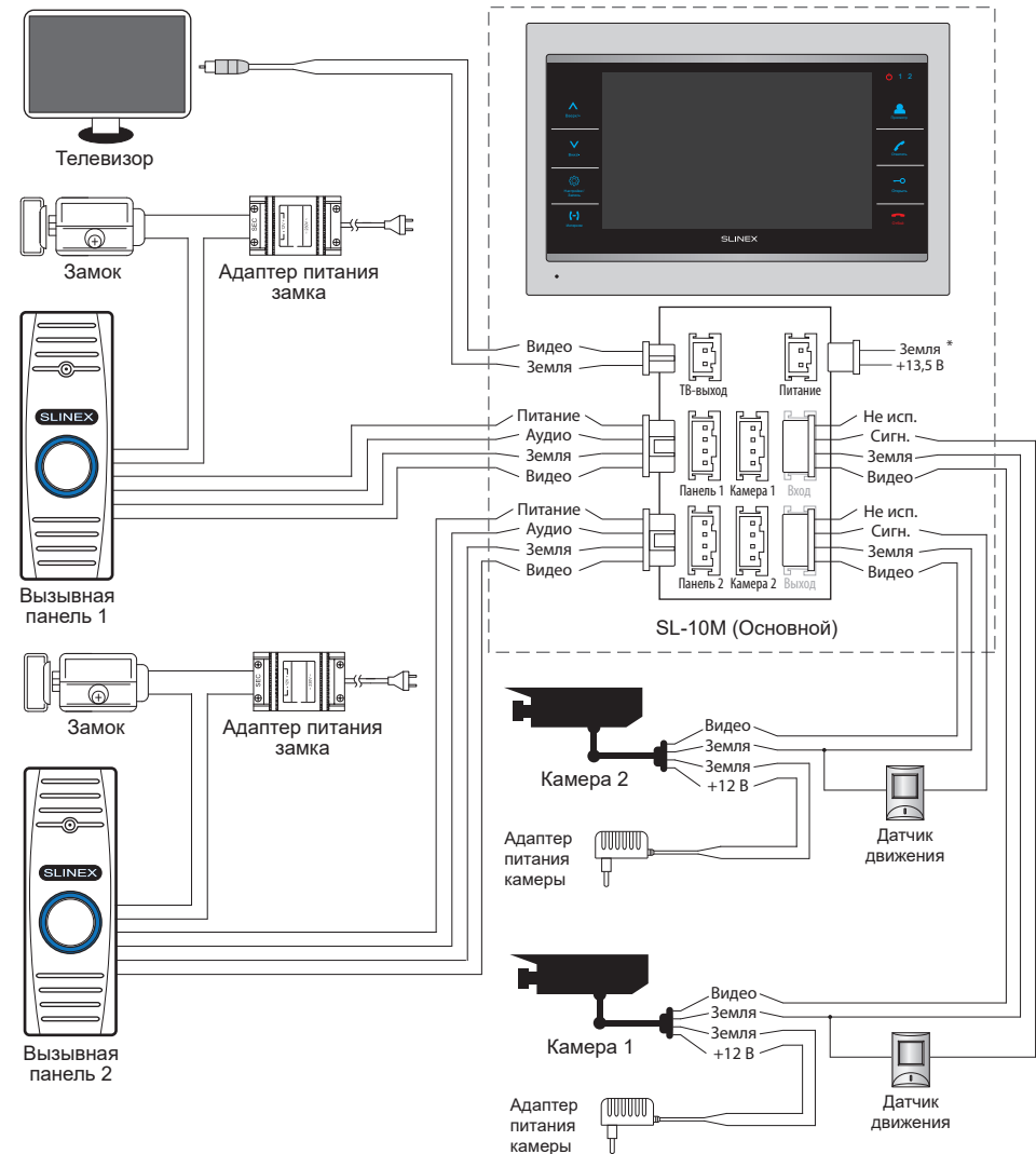
Схема 1. Подключение вызывных панелей, камер и телевизора к домофону SL-10M.
