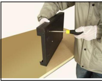
4. закрепите жесткий диск
