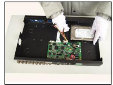
6. подключите кабель питания
