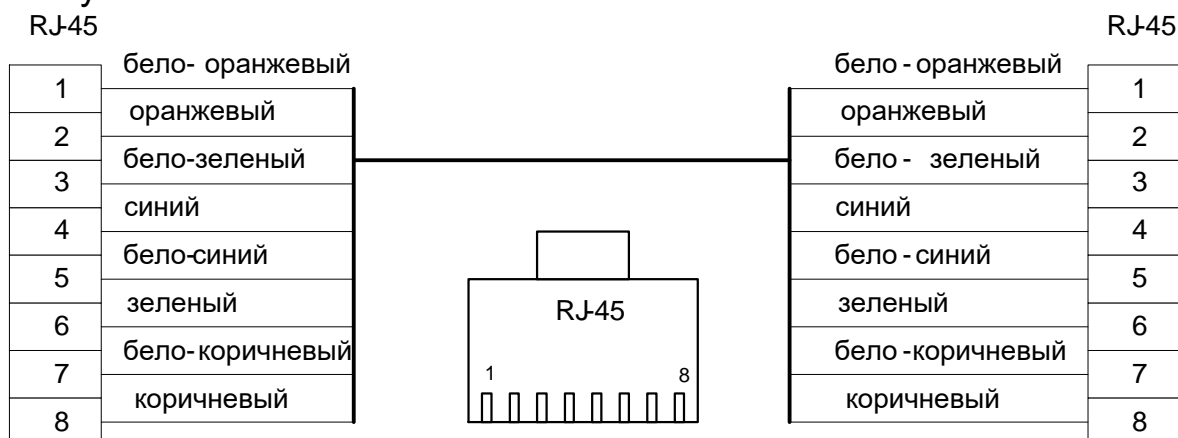
Рис. 6.4. Разделка кабеля.
