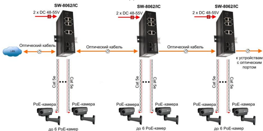
Рис.4 Типовая схема подключения коммутатора SW-8062/IC
