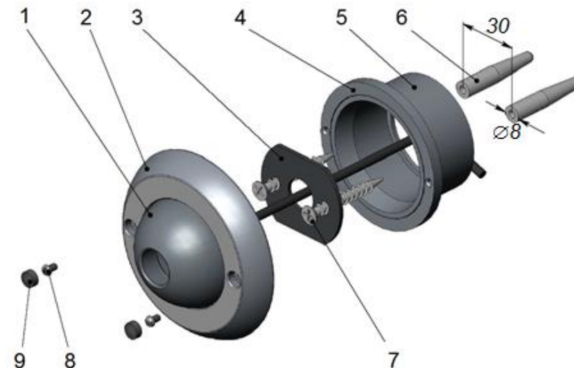
1 - видеокамера-шар; 2 - накладка; 3 - дно; 4 – фланец; 5 – гильза; 6 – дюбель; 7 - шуруп; 8 – винт М3х8; 9.- заглушка.
